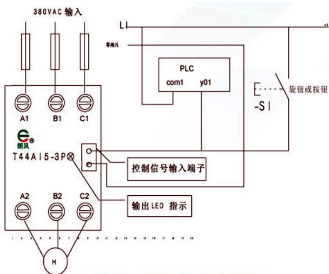
朗风无触点A系列接线示意图
