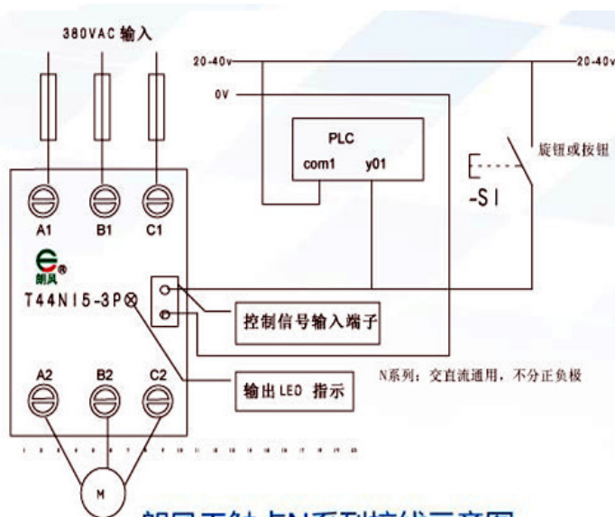
朗风无触点N系列接线示意图
